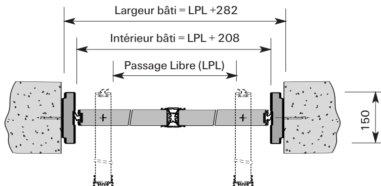
Coupe horizontale
