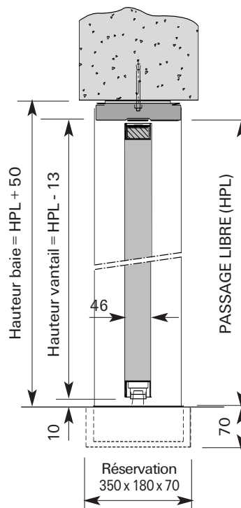
Coupe verticale
