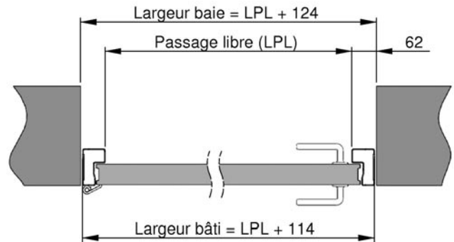
Coupe horizontale
