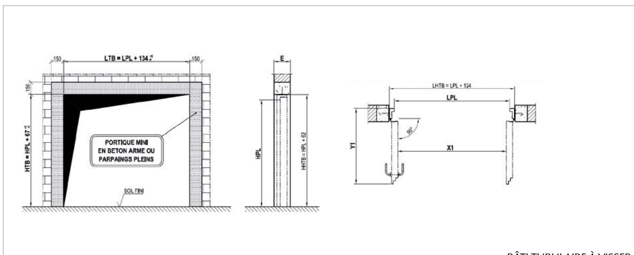
BÂTI TUBULAIRE À VISSER
