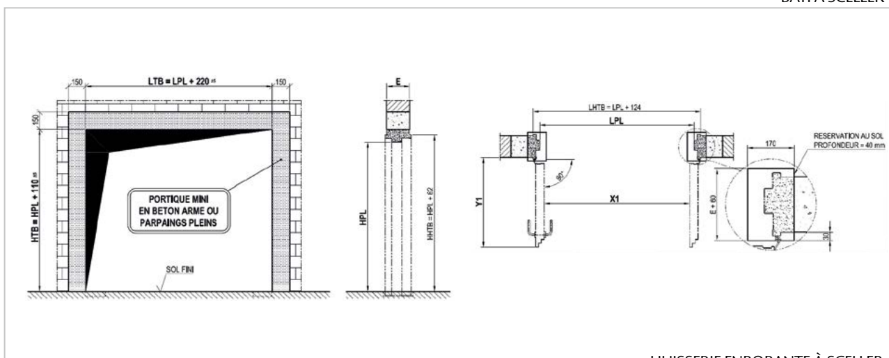
HUISSERIE ENROBANTE À SCELLER
