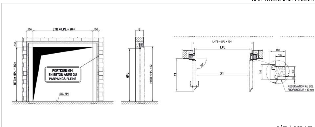
BÂTI À SCELLER
