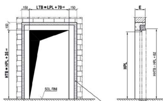
PORTIQUE MINI EN BETON ARME OU PARPAINGS PLEINS
