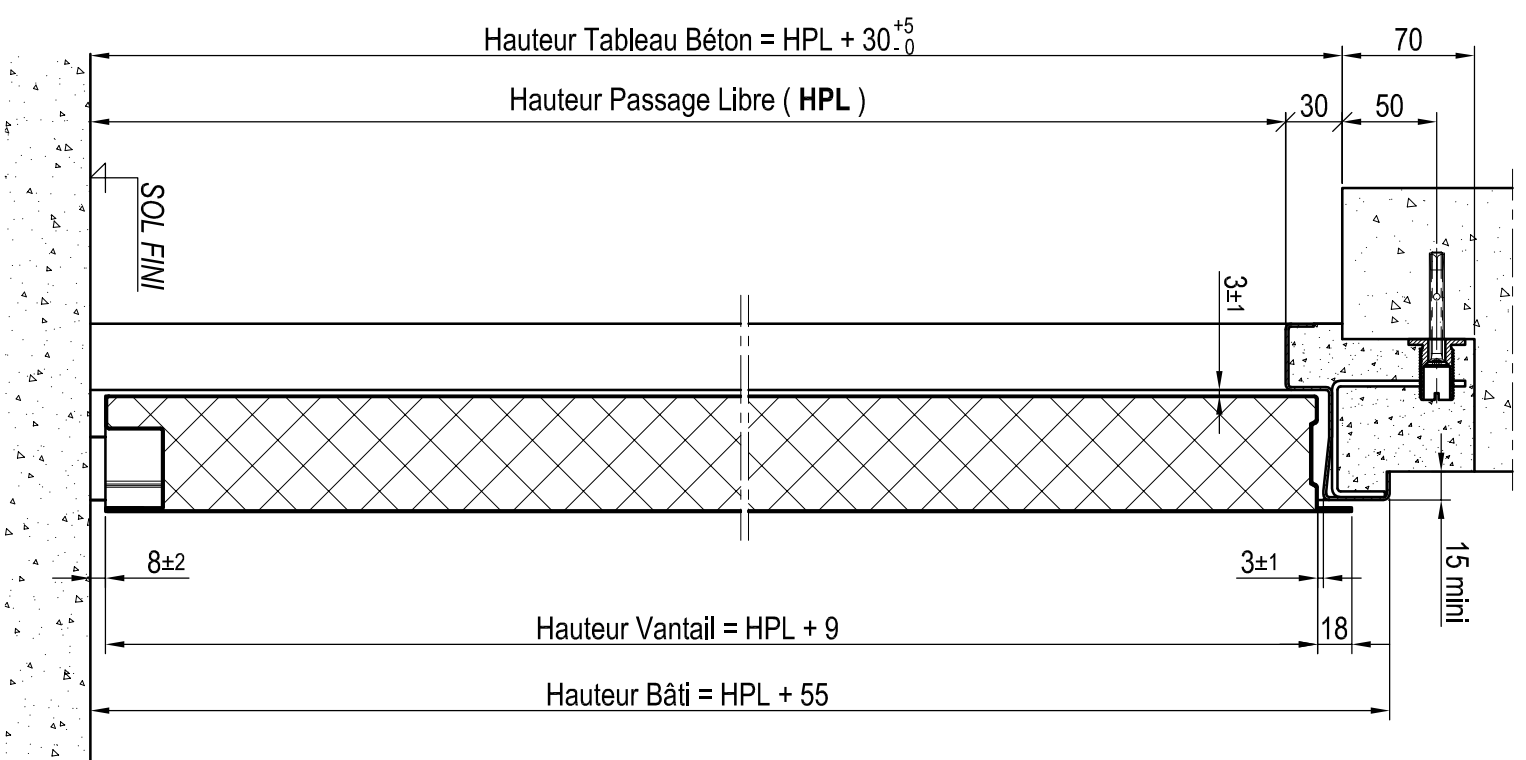
COUPE VERTICALE
